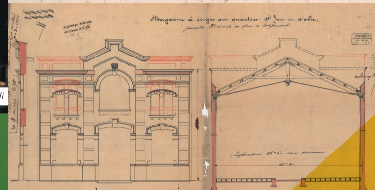
21. Bouwplan van het pakhuis, 1895 © Archief Gent
